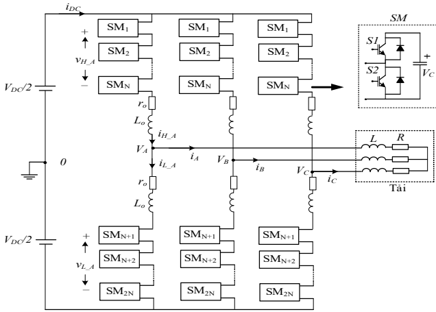
Hình 1. Cấu trúc bộ biến đổi MMC
