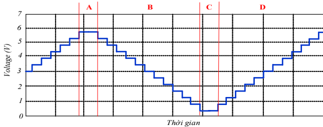
Hình 5. Trạng thái điện áp AC đầu ra của bộ MMC
