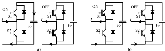
Hình 2. Trạng thái ON và OFF của các SM khi:
