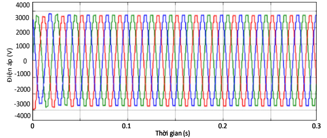
Hình 7. Điện áp ba pha phía xoay chiều
