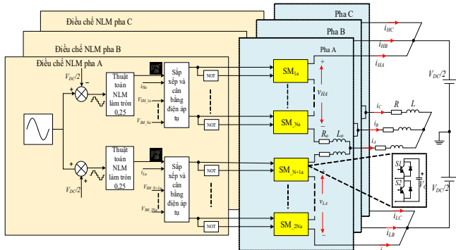
Hình 6. Cấu trúc điều chế NLM cải tiến kết hợp với cân bằng điện áp tụ điện cho BBD MMC
