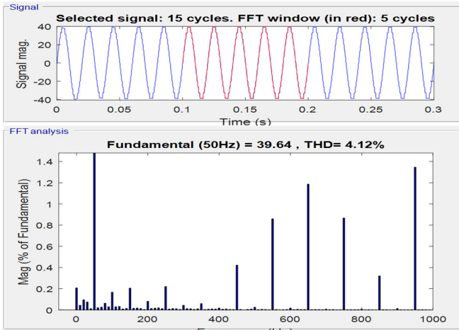
Hình 10. Kết quả phân tích Fourier dòng điện
