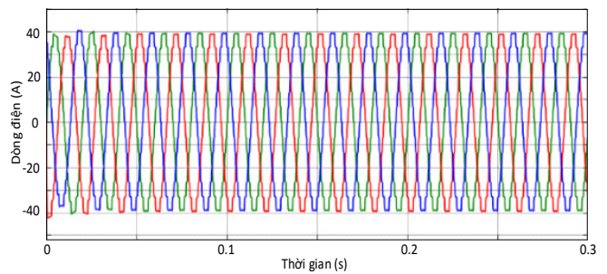
Hình 8. Dòng điện ba pha phía xoay chiều cung cấp cho tải
