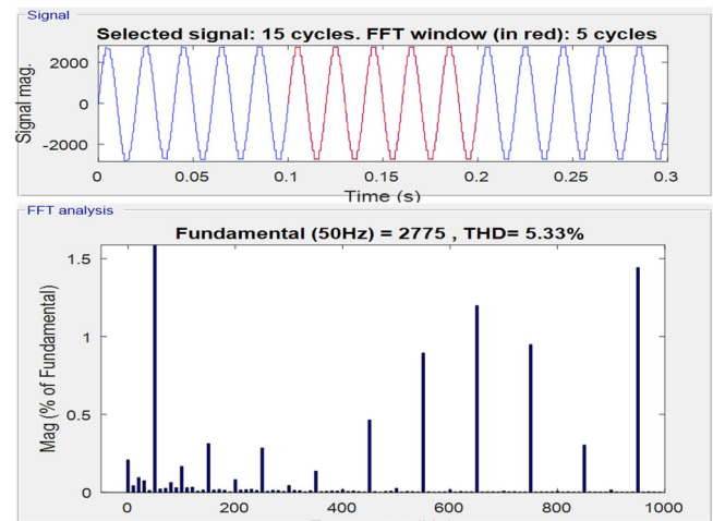
Hình 9. Kết quả phân tích Fourier điện áp
