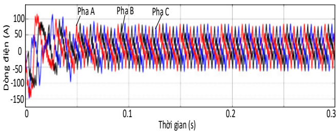
Hình 12. Dòng điện vòng trong các pha của MMC
