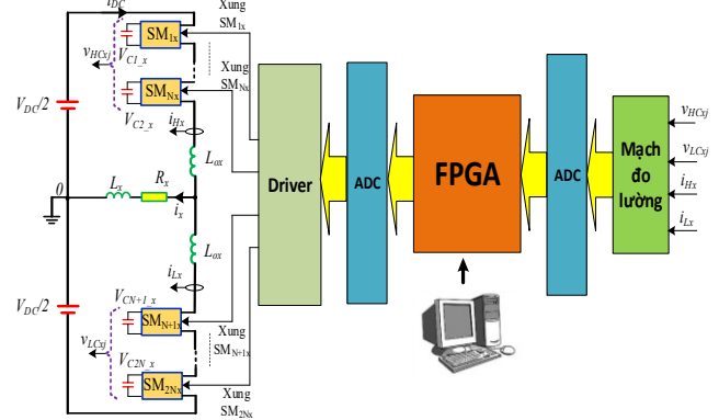
Hình 13. Cấu trúc hệ thống thực nghiệm một pha của MMC
