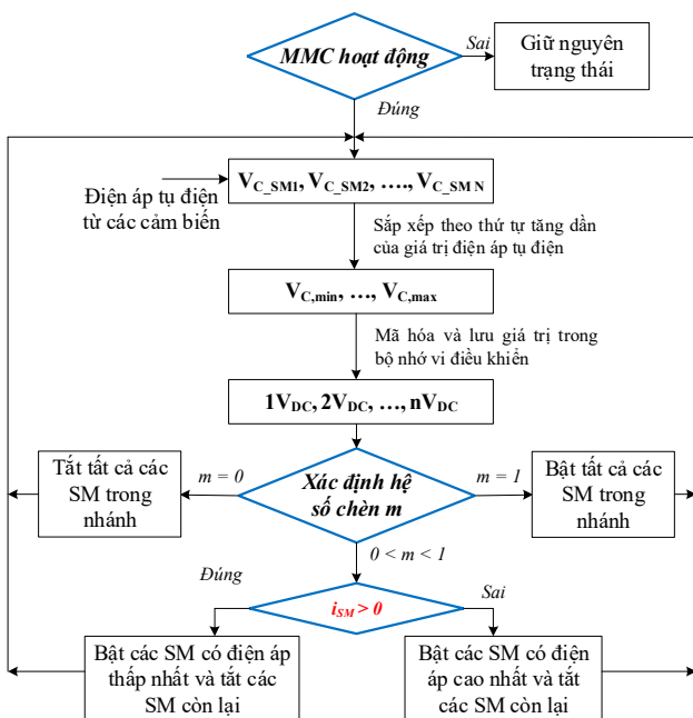
Hình 4. Lưu đồ thuật toán cân bằng điện áp tụ điện
