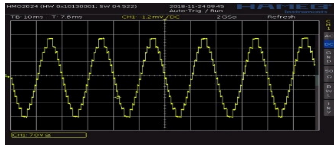
Hình 15. Điện áp trên tải xoay chiều
