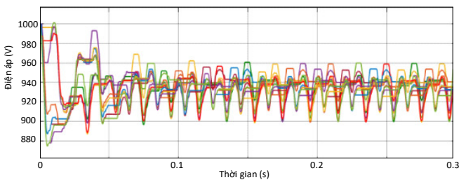
Hình 11. Điện áp các tụ điện của nhánh trên và dưới pha A
