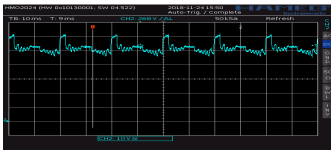
Hình 17. Điện áp trên tụ điện của SM1
